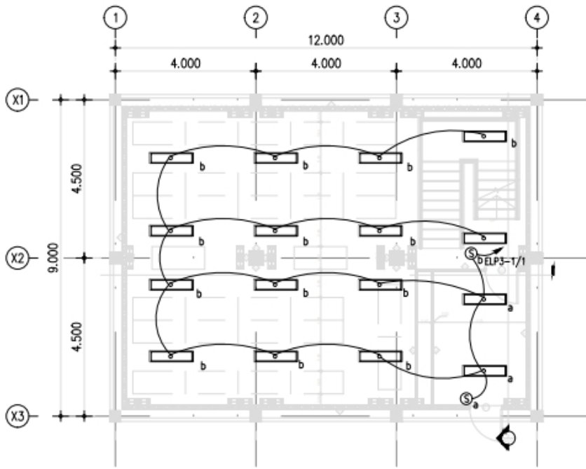
ผังพื้นชั้น 3 SCALE A3-11100
