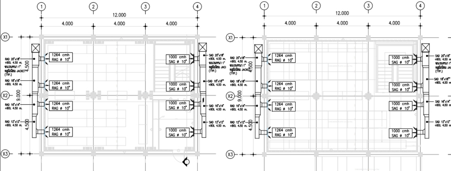
ผังพื้นที่ 3 SCALE A3-1:1100
