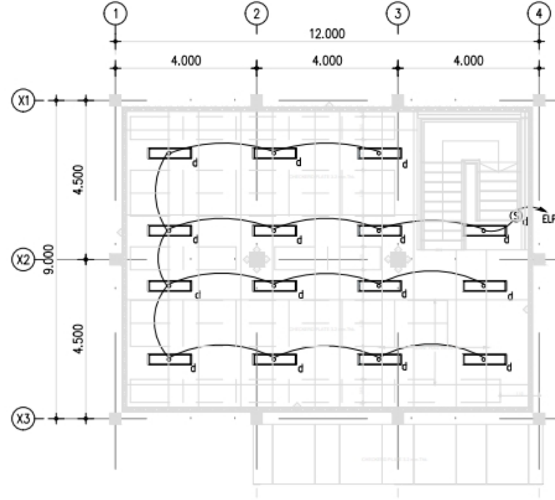
ผังพื้นชั้น 3/ลอย SCALE A3-11100
