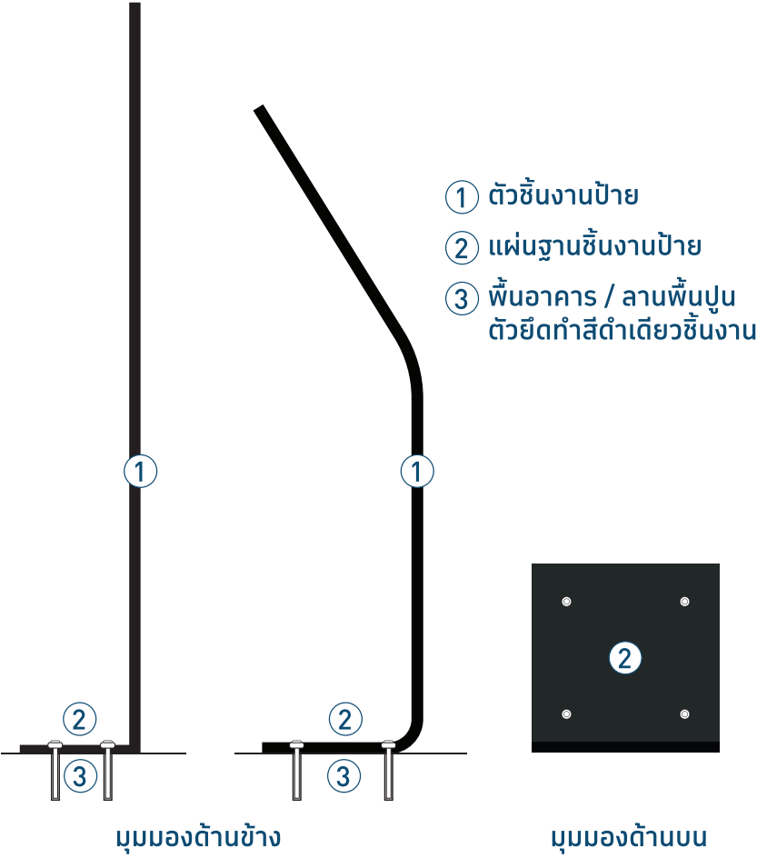
แบบยึดฐานกับพื้น
