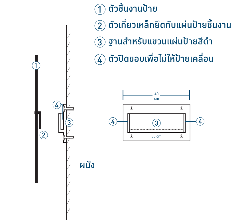
มุมมองด้านข้าง
